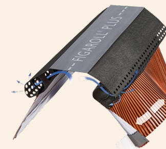
Taśma Figaroll właściwa wentylacja w obrębie kalenicy
